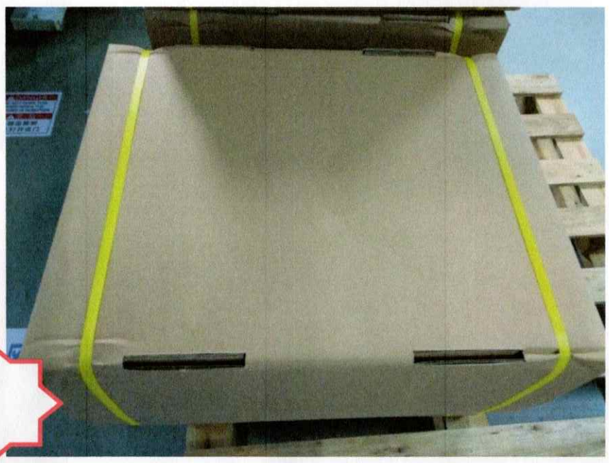
图二，确认 PA3215 无漏装后，将 26 的内箱与外箱配合并打包装带待出货
